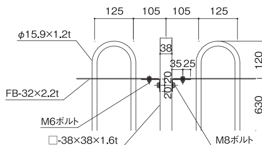
支柱納まり部詳細(スケール1/6)
