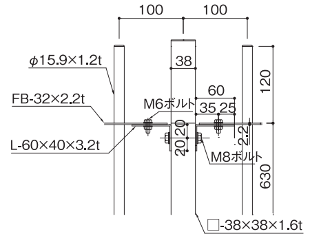
支柱納り部 詳細(スケール1/4)
