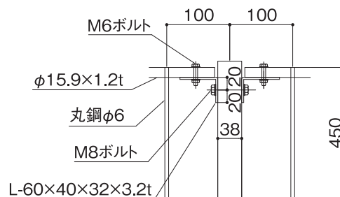
支柱納まり部詳細(スケール1/5)
