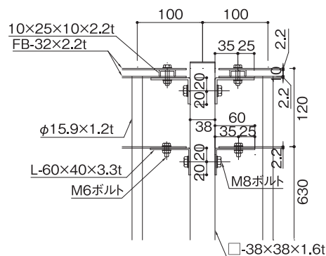
支柱納り部 詳細(スケール1/4)
