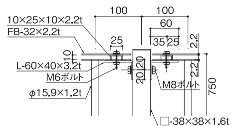
支柱納り部 詳細(スケール1/4)
